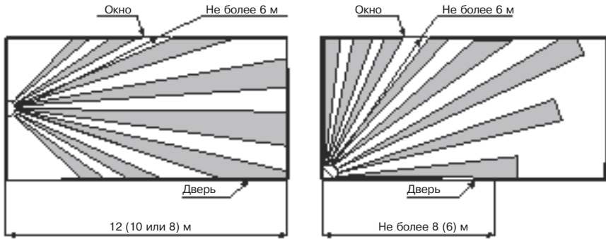
Рисунок В.1 – Установка извещателей «Орлан» и «Орлан-Д» на стене и в углу помещения (длина помещения не более 12 м для извещателя «Орлан»; 10 или 8 м для извещателя «Ор-лан-Д»)
