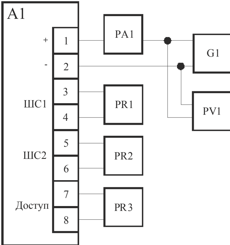
Схема соединений для проверки извещателя
