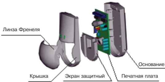
Рисунок Б.5 – Составные части извещателя
